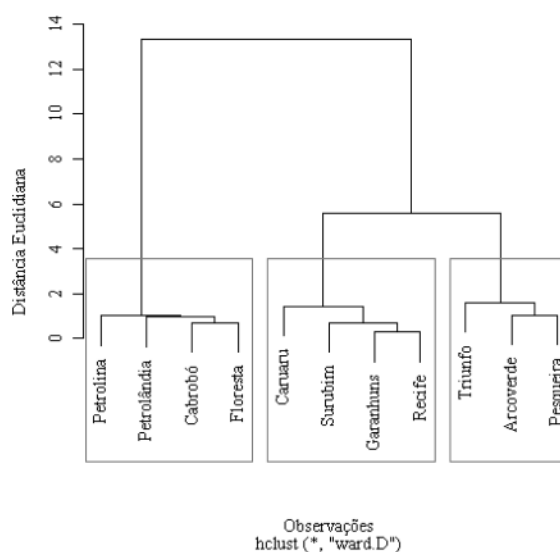
Figura 2. Dendograma com análise de agrupamento ( clusters ) aplicado à distância Euclidiana pelo método de Ward para os 11 municípios, em função da análise de precipitação pluvial de 1961 a 1990. Grupo 1: Petrolina, Petrolândia, Cabrobó e Floresta; Grupo 2: Caruaru, Surubim, Garanhuns e Recife; Grupo 3: Triunfo, Arcoverde e Pesqueira.
