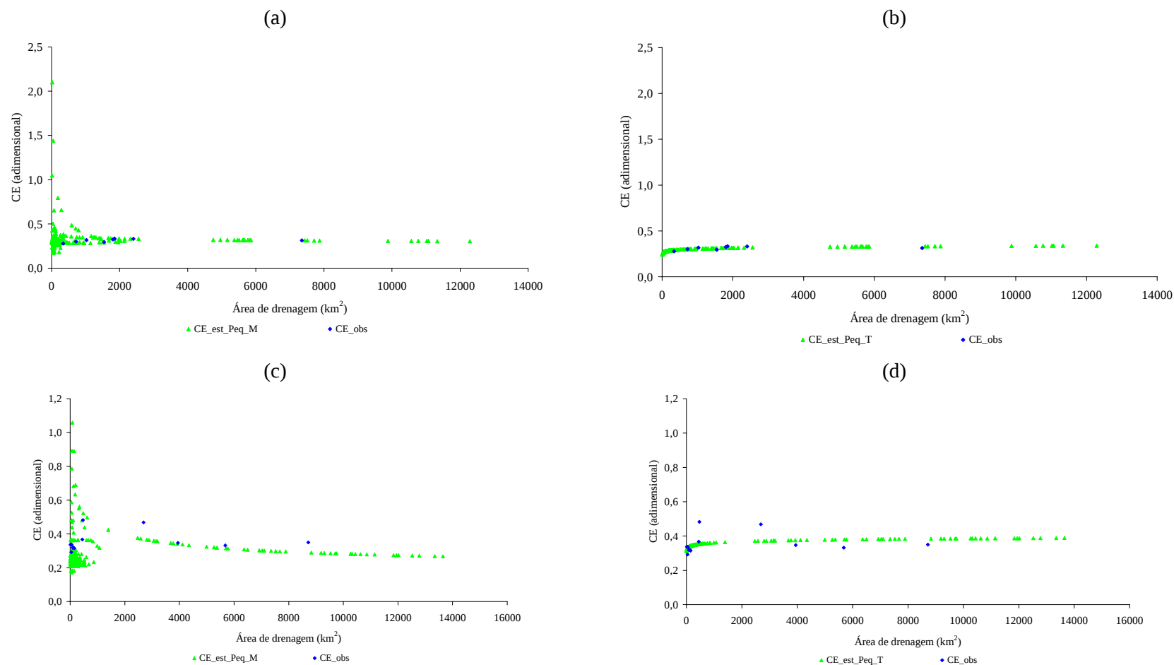
Figura 1C – Coeficientes de escoamento superficial obtidos com base nas vazões estimadas em função da P_{\text{eq}} pelo MCM (a); e pelo método tradicional (b) em cada trecho da base hidrográfica da bacia do rio Pará e Paraopeba, respectivamente e os observados em suas estações.
